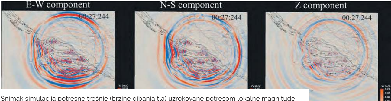
Snimak simulacija potresne trešnje (brzine gibanja tla) uzrokovane potresom lokalne magnitude 6.1 kod Makarske 1962. godine
