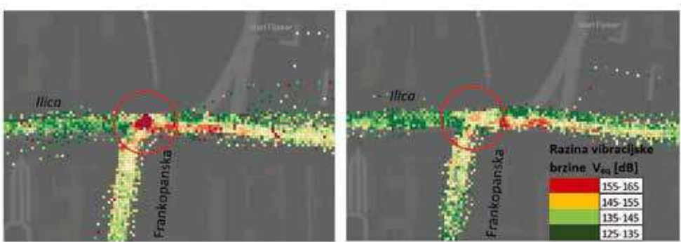
SLIKA 4 :Prikaz smanjenja razina vibracija izmjerenih na tramvajskom vozilu na raskrižju Frankopanska – Ilica prije (lijevo) i nakon zamjenekrižališta (desno)
