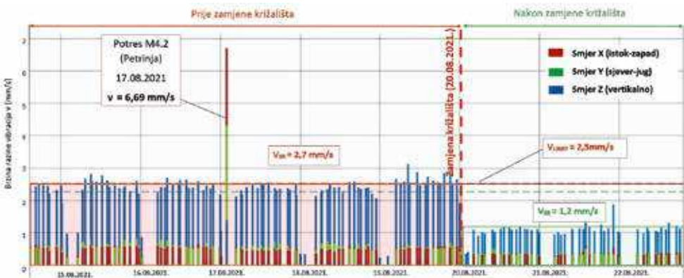
SLIKA 6: Prikaz razina vibracija izmjerenih na zgradama prije i nakon intervencije na kolosijeku na raskrižju Ilica – Frankopanska
